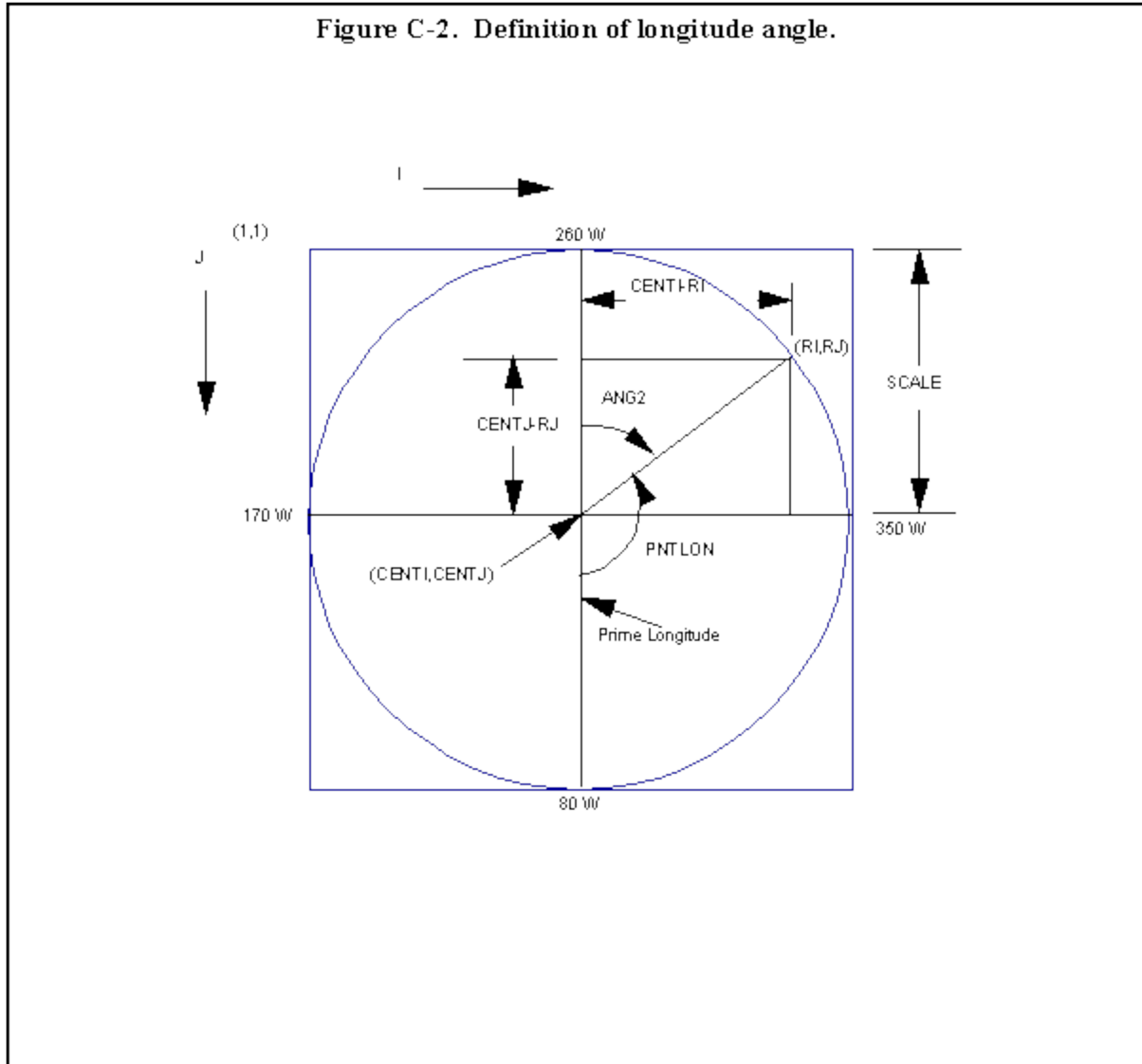
Figure C-2. Definition of longitude angle.
